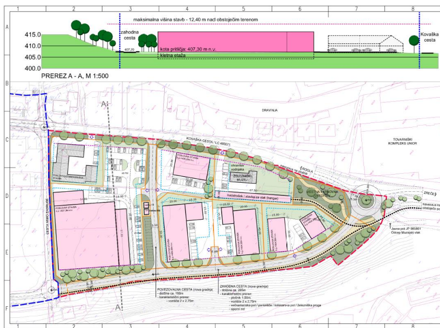
Slika 39: Ureditvena situacija poslovno-obrtne cone Zreče
