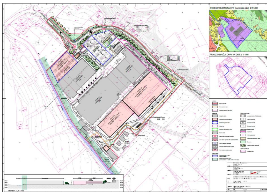
Slika 42: Ureditvena situacija OPPN Spodnja industrijska cona Zreče
