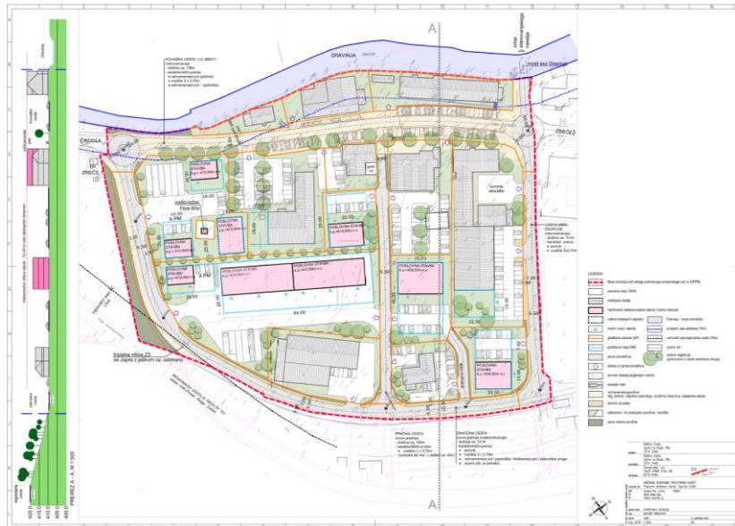
Slika 38: Ureditvena situacija za območje poslovne zazidave Zgornje Zreče
