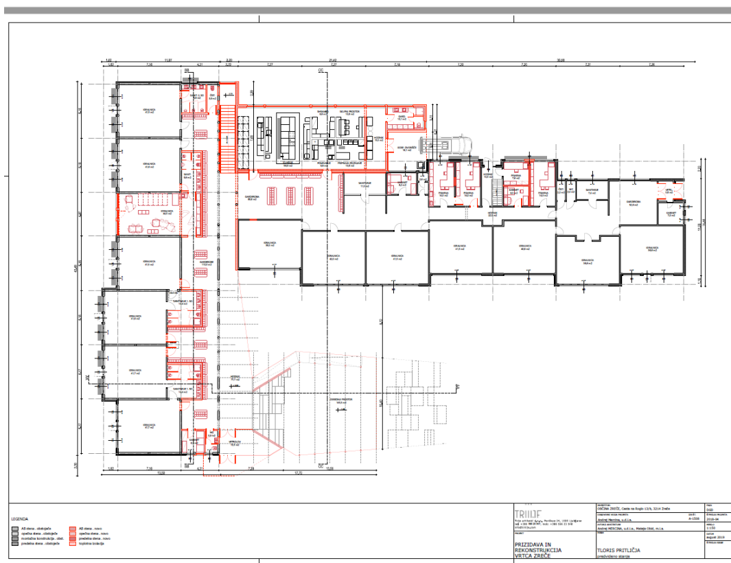
Slika 62: Načrt izgradnje kuhinje Vrtca Zreče
