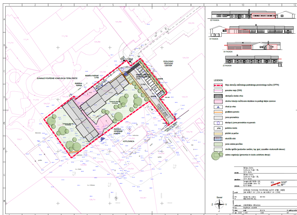
Slika 41: Ureditvena situacija OPPN Vrtec Zreče
